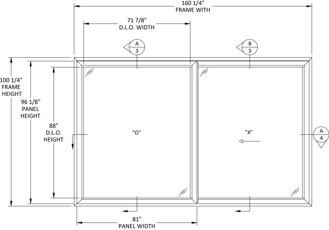
ELEVATION
